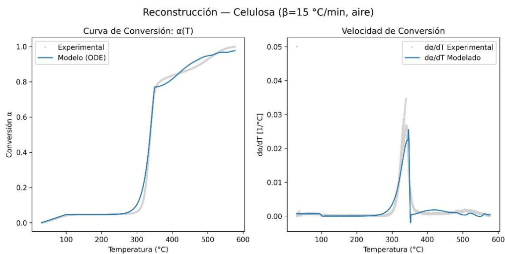
Figura 1. Curvas TGA experimental (gris) y modelada (azul).
